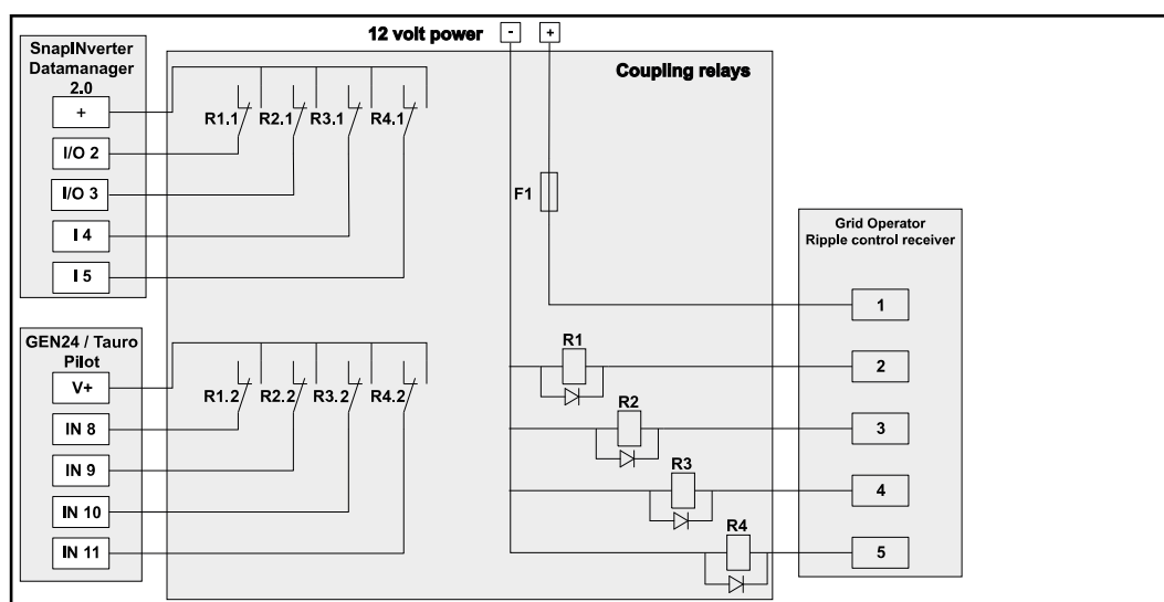
Anschluss-Schema Rundsteuer-Empfänger mit mehreren Wechselrichtern
